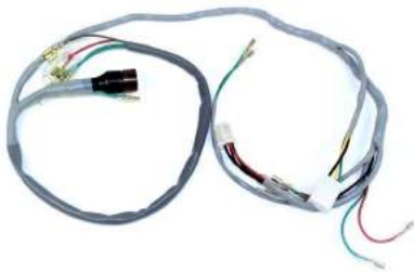
CT70K0 Wire Harness CT70 K0 DAX
